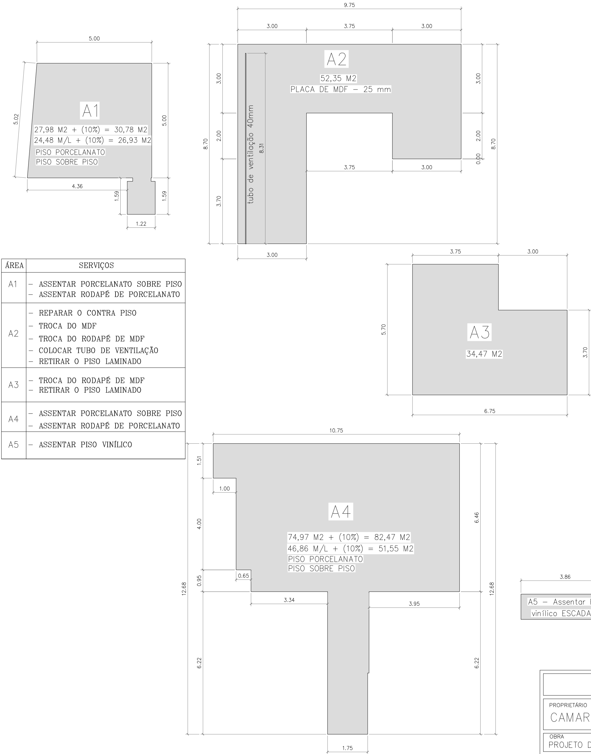
LAYOUT (ÁREA A SER REFORMADA) ESCALA: 1:100
