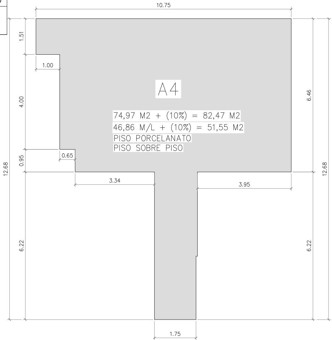
LAYOUT (ÁREA A SER REFORMADA) ESCALA: 1:100
